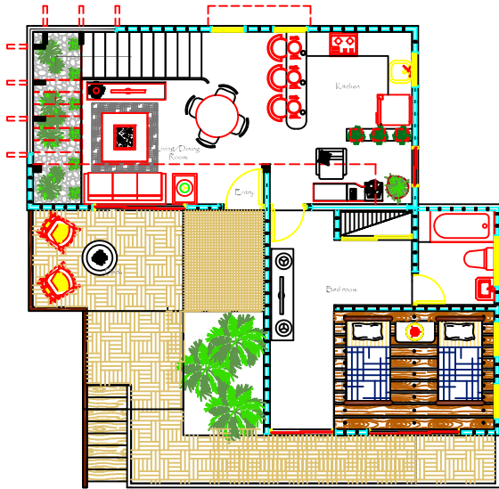
PLANTA ARQ. 1er NIVEL
