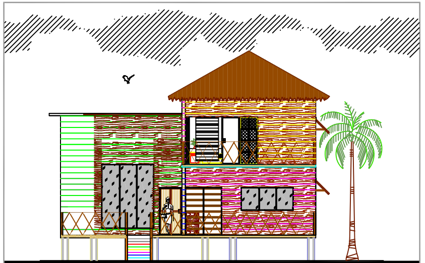
ELEVACION FRONTAL
