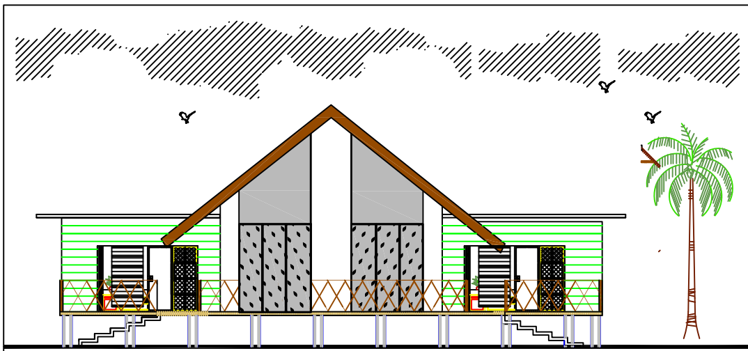
ELEVACION FRONTAL
